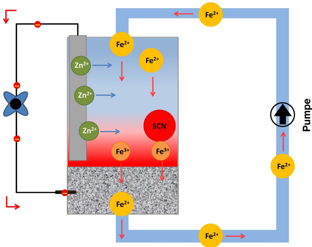
Abb. 16: Schematische Darstellung des Entladevorgangs der Freiburger Hybrid-Redox-Flow-Batterie auf Basis von elementarem Zink und einer \text{Fe}^{3+} -Lösung im Med-Tec-Ansatz.
