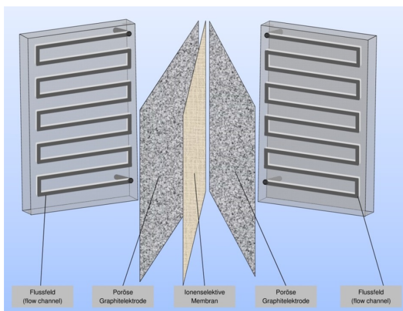
Abb. 3: Aufbau eines brennstoffzellenähnlichen Energiewandlers einer Redox-Flow-Batterie.
