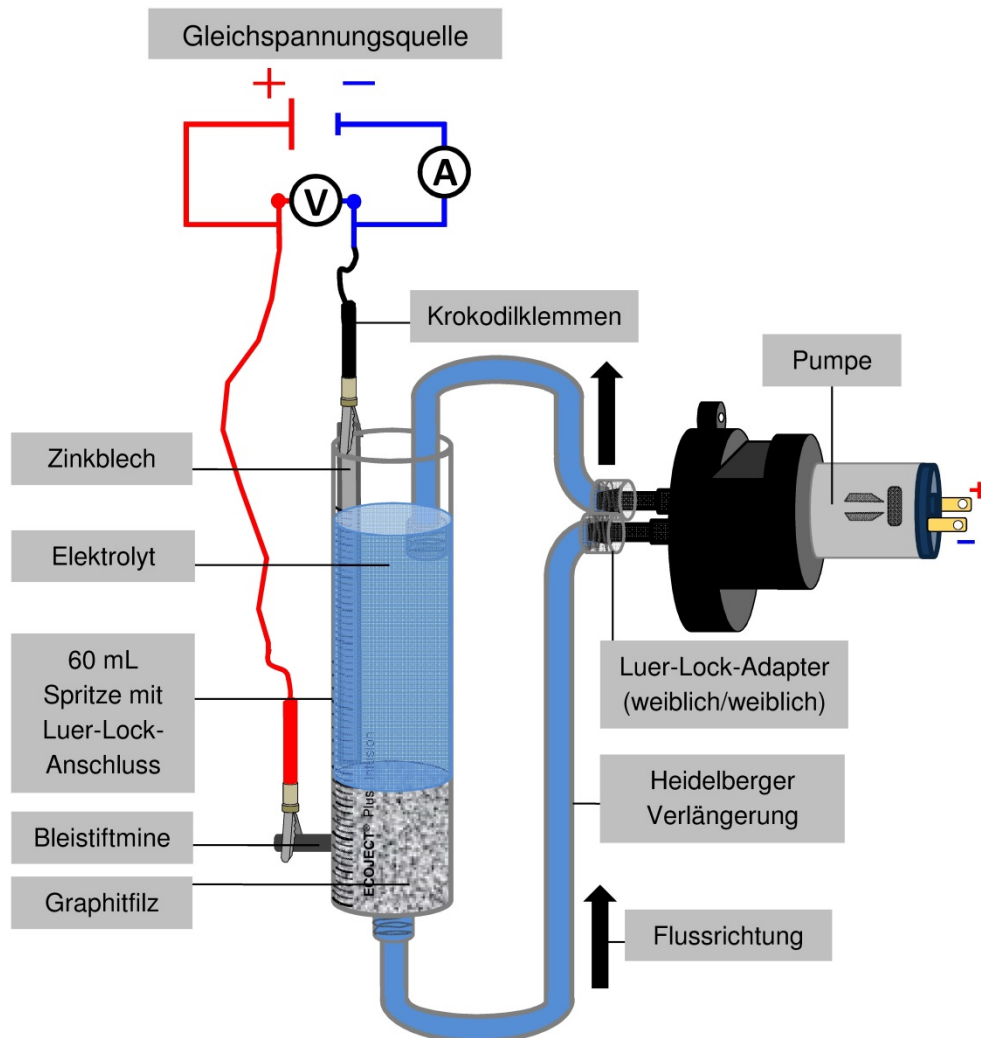
Abb. 11: Schematische Darstellung des Versuchsaufbaus der Freiburger Hybrid-Redox-Flow-Batterie im Med-Tec-Ansatz.
