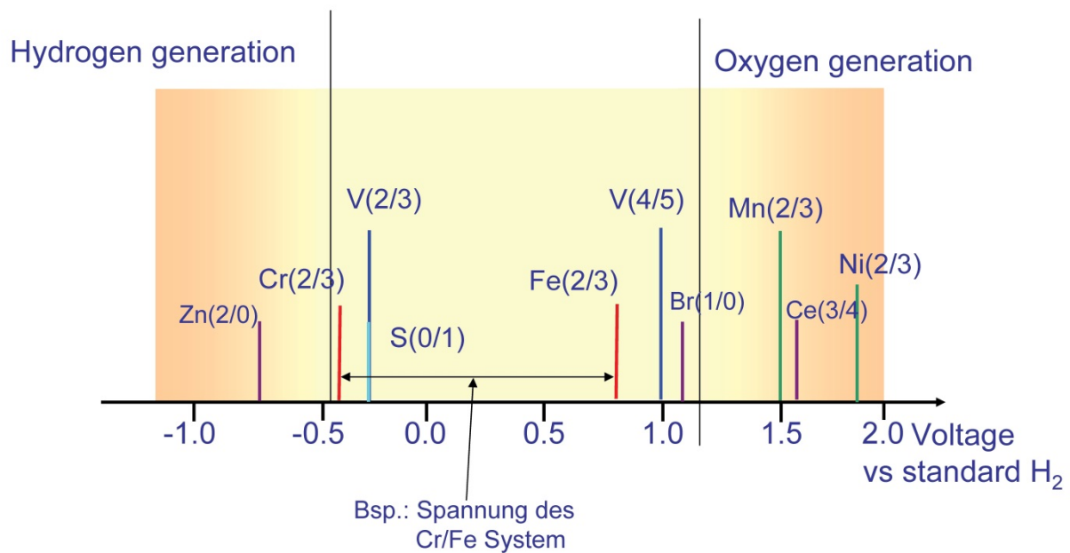
Abb. 7: Einige mögliche Redoxpaare in Redox-Flow-Batterien und deren Standardelektrodenpotentiale. Die zueinander gehörenden Paare wurden farblich identisch gekennzeichnet.
