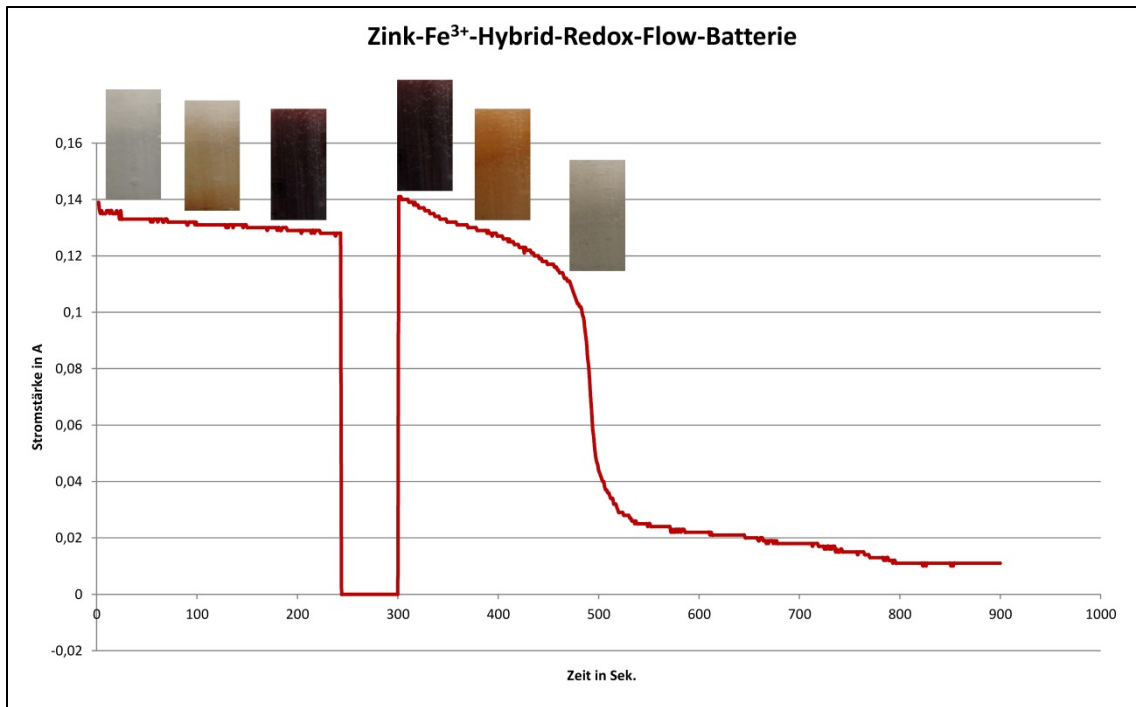
Abb. 14: Strom/Zeit-Diagramm mit Färbung während des Lade- und Entladevorgangs der Freiburger Hybrid-Redox-Flow-Batterie auf Basis von metallischem Zink und einer Fe 3+ -Lösung.
