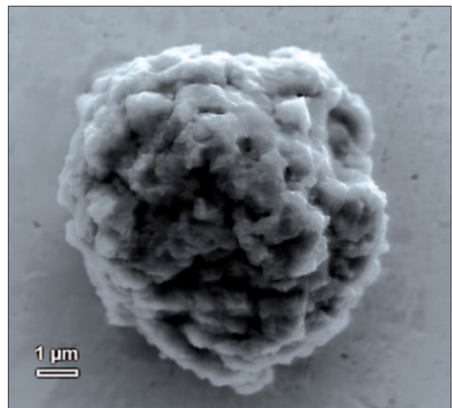
Sternenstaub von Roten Riesen – Siliziumkarbid-Korn aus dem Meteoriten Murchison. (© J. Huth, S. Merchel, MPI Mainz)
