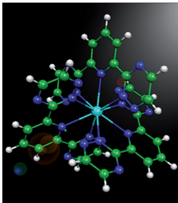
Komplex des dreiwertigen Americiumions mit drei Bis-Triazinyl-Pyridin-Molekülen. Dabei handelt es sich um ein hochselektives Extraktionsreagenz für die Actiniden-Lanthanidentrennung. (© KIT)
