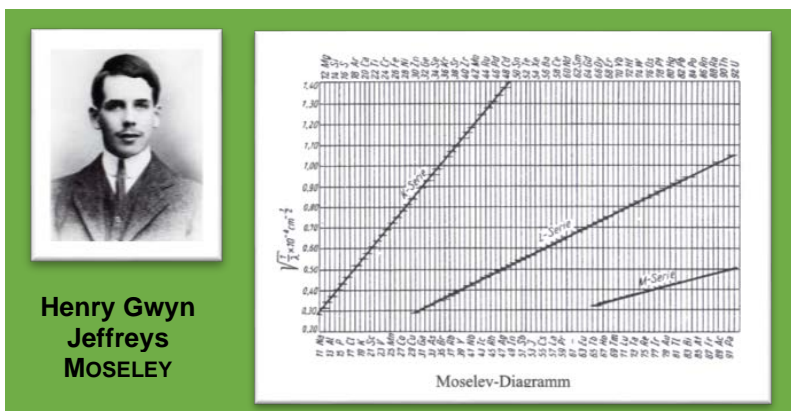
Abb. 16. MOSELEYS Entdeckung der Kernladungszahl der Elemente als Ordnungsprinzip im Periodensystem der Elemente
