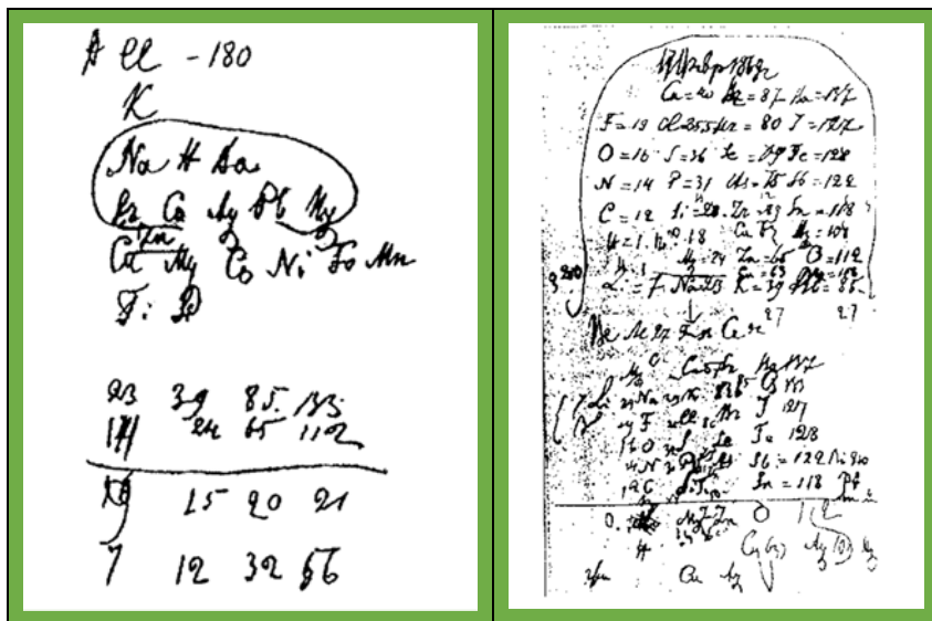
Abb. 7. Links: Notizen MENDELEJEWS auf der Rückseite des Briefes von CHODNEW; Rechts: Notizen MENDELEJEWS auf der Rückseite des Briefes vom FOG-Vorstand 15)
