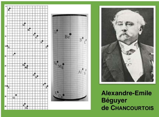
Abb. 4. de CHANCOURTOIS' Anordnung der damals bekannten chemischen Elemente in der Reihenfolge ihrer Atomgewichte auf einer tellurischen Helix oder tellurischen Schraube
