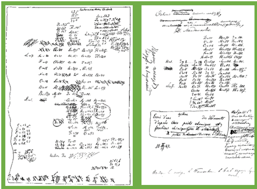
Abb. 8. Links: Notizen MENDELEJEWS nach dem „chemischen Patience-Spiel“ mit Elementkärtchen; Rechts: MENDELEJEWS Manuskript des ins reine aufgeschriebenen Periodensystems 13)
