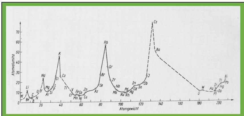
Abb. 11. Die Periodizität der Atomvolumina in Abhängigkeit von den Atomgewichten nach MEYER 21)
